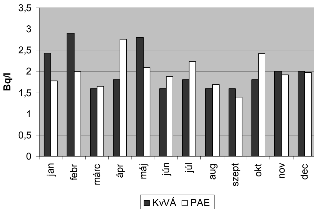
2.5.b.ábra. A melegvíz csatorna (V2) trícium-koncentrációjának havi átlagértékei Figure 2.5.b. Monthly tritium concentrations in the hot water (discharge) channel (KVvÁ: measured by SEW; PAE: measured by NPP)
