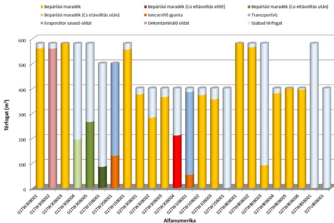
3.1. ábra. A folyékony hulladéktároló tartályok töltöttsége (2012. decemberi állapot) Figure 3.1. The used volumes of the liquid waste storage tanks on December 2012
