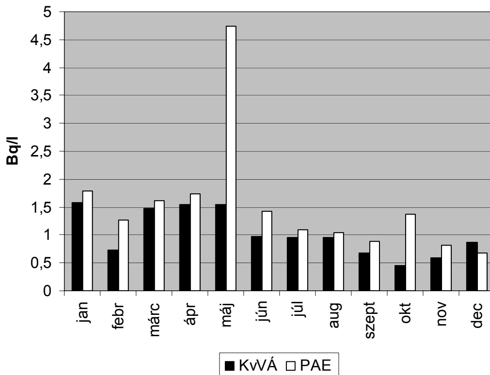
2.4.c. ábra. A szennyvíz csatorna (V3) összes-béta aktivitáskonzentrációjának havi átlagértékei Figure 2.4.c. Monthly gross beta activity concentration in the waste water channel (KWÁ: measured by SEW; PAE: measured by NPP)
