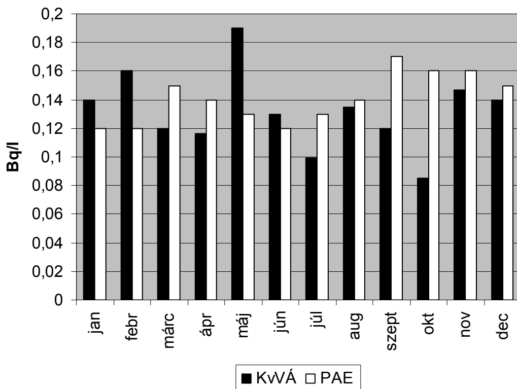
2.4.b. ábra. A melegvíz csatorna (V2) összes-béta aktivitáskonzentrációjának havi átlagértékei Figure 2.4.b. Monthly gross beta activity concentration in the hot water (discharge) channel (KVvÁ: measured by SEW; PAE: measured by NPP)
