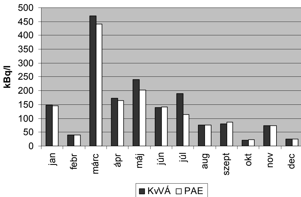
2.5.c.ábra. A szennyvíz csatorna (V3) trícium koncentrációjának havi átlagértékei Figure 2.5.c. Monthly tritium concentrations in the waste water channel (KVvÁ: measured by SEW; PAE: measured by NPP)
