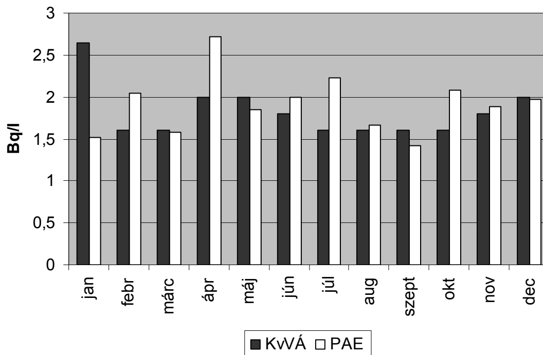
2.5.a. ábra. A hidegvíz csatorna (V1) trícium koncentrációjának havi átlagértékei Figure 2.5.a. Monthly tritium concentrations in the inflow water channel (KWÁ: measured by SEW; PAE: measured by NPP)
