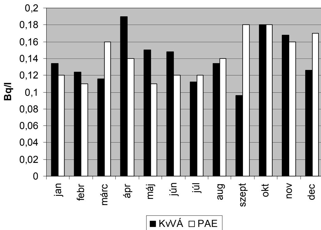
2.4.a. ábra. A hidegvíz csatorna (V1) összes-béta aktivitáskonzentrációjának havi átlagértékei Figure 2.4.a. Monthly gross beta activity concentration in the inflow water channel (KVvÁ: measured by SEW; PAE: measured by NPP)
